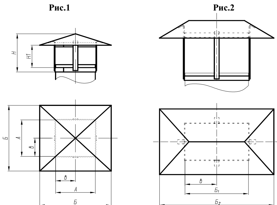
Рисунок 4.2 Зонты прямоугольные ЗПц
