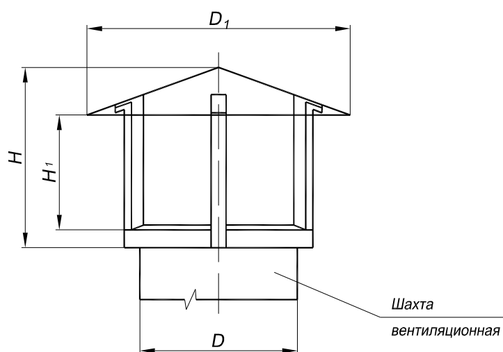
Рисунок 4.1 Зонты круглые ЗКц
